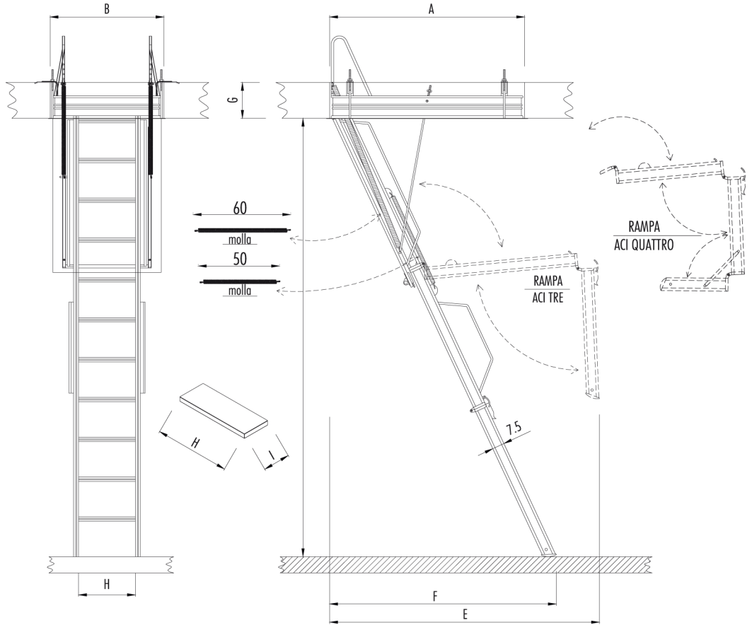
Aletta del corpo cassonetto 3cm. Frame's width
